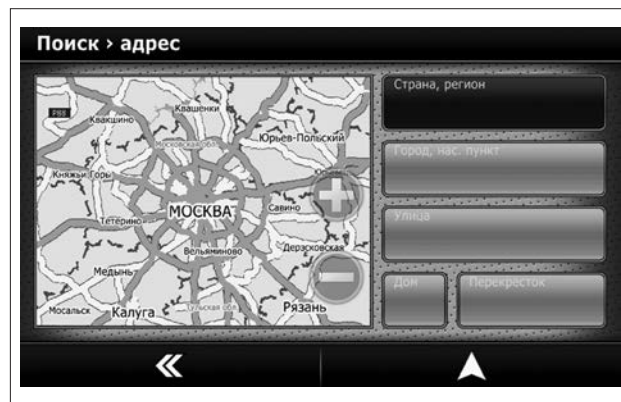
Рис. 26. Выбор адреса
