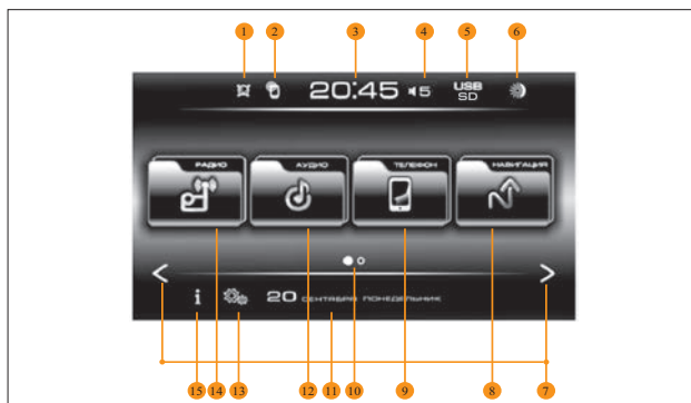
Рис. 3. Главное меню
