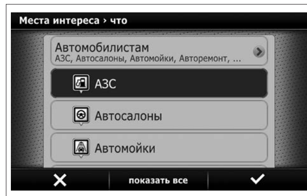
Рис. 42. Выбор подкатеории
