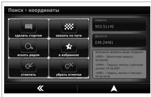
Рис. 52. Дополнительное меню
