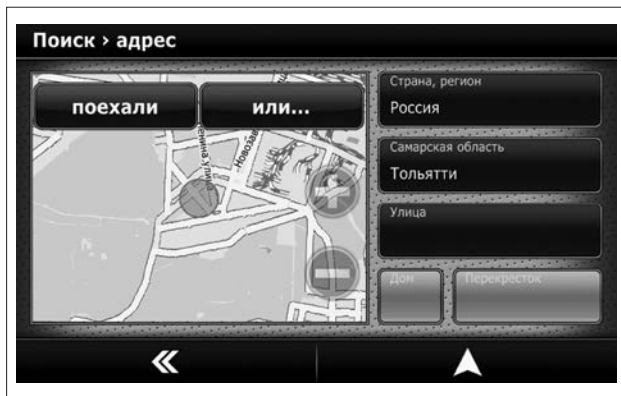
Рис. 31. Поиск улицы
